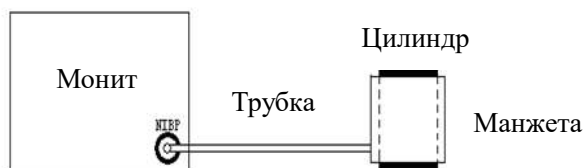
Рис. 23-1. Схема подключения для теста утечки НИАД
