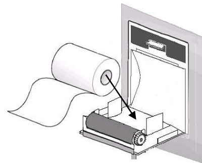
Рис. 18-2. Установка бумаги для печати
