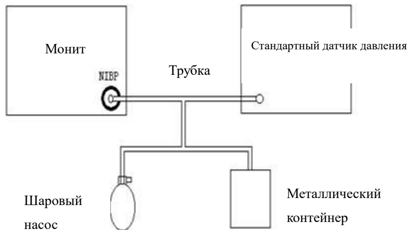
Рис. 23-2. Схема подключения для проверки НИАД
