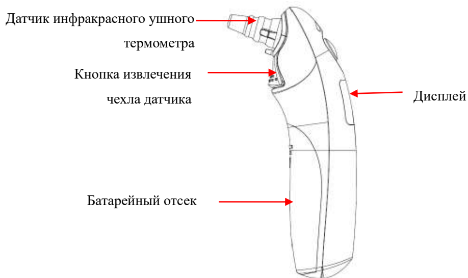
Рис. 14-2. Инфракрасный ушной термометр: вид сбоку
