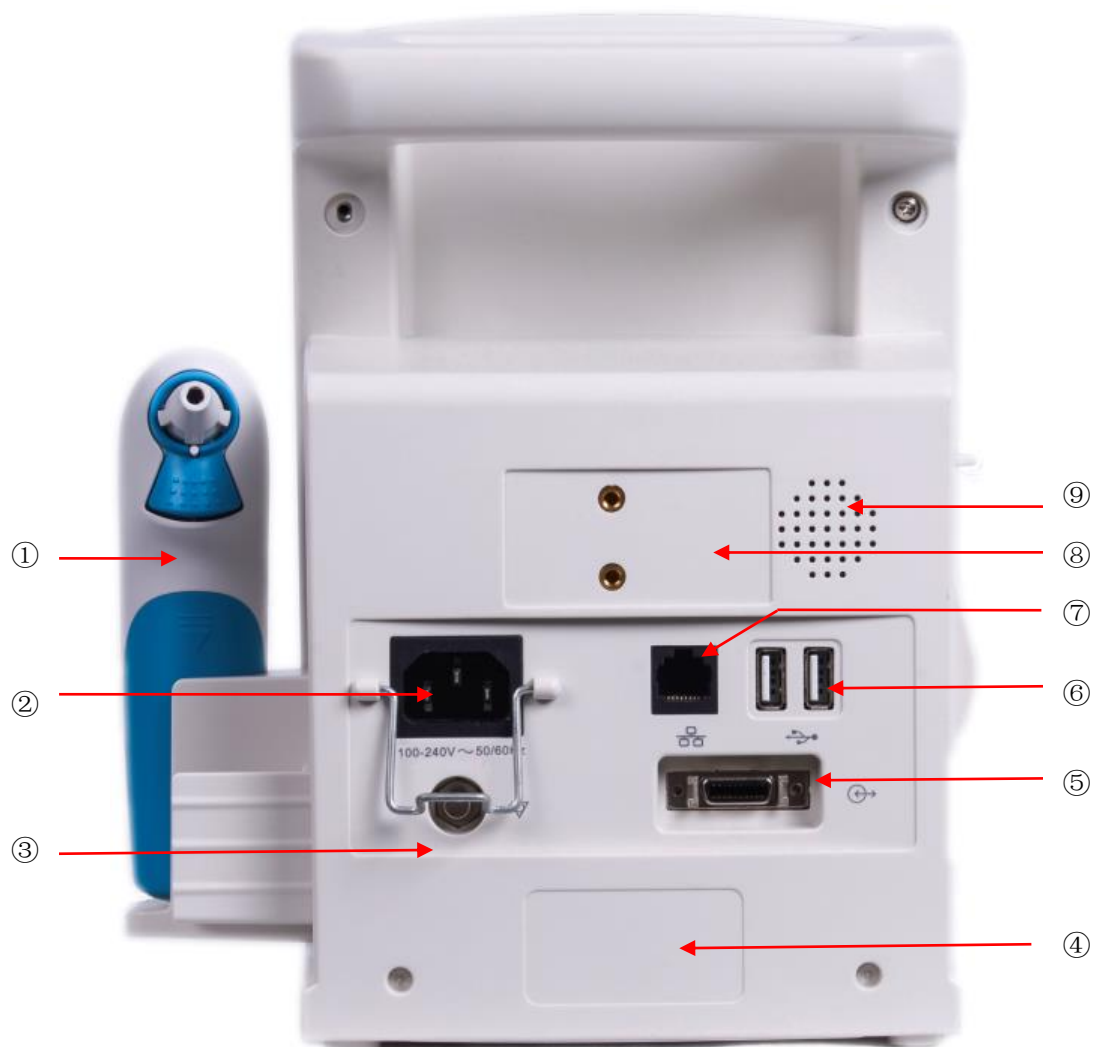
Рис. 2-4. Задняя крышка
