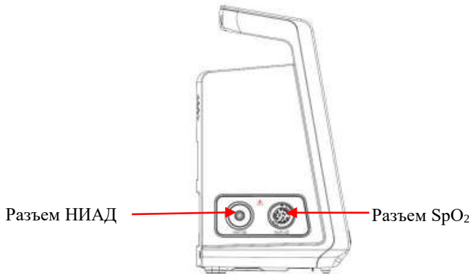
Рис. 2-2. Левая панель
