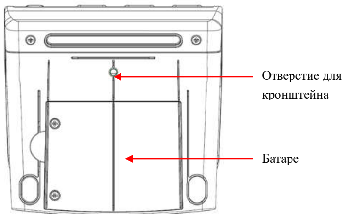
Рис. 2.5. Крышка основы
