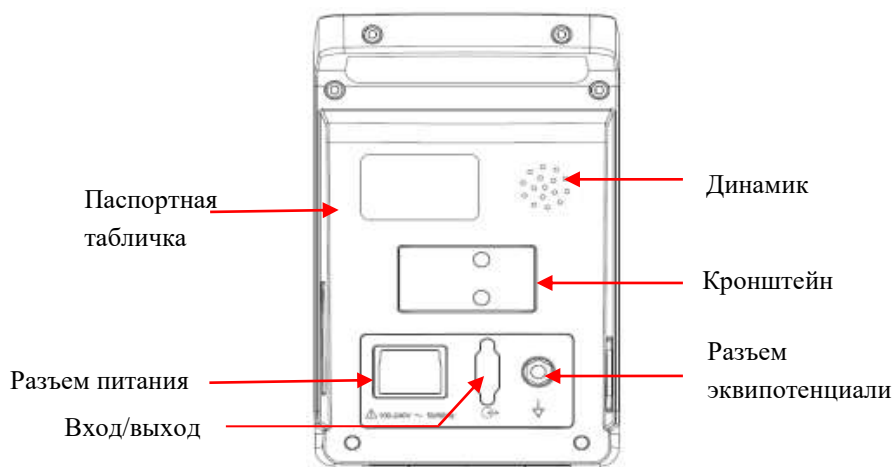
Рис. 2- 4. Задняя панель
