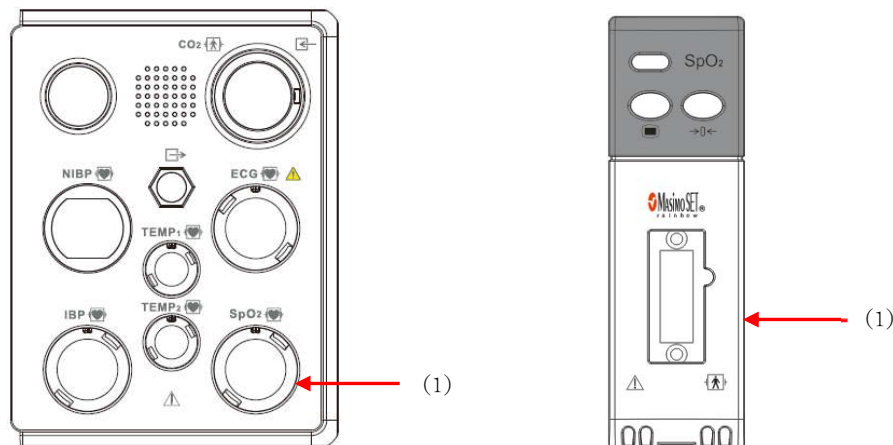
(1) Разъем кабеля SpO2
