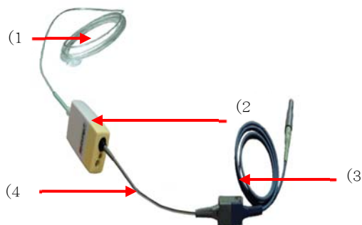
(1) Линия отбора проб (2) Датчик CO 2 (3) Соединительный кабель "Масимо" (4) Кабель датчика
